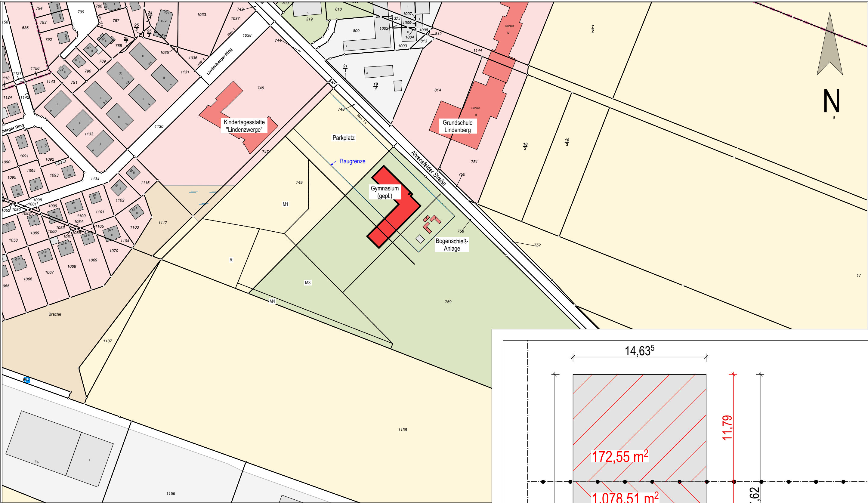
Auszug aus Liegenschaftskarte mit Projekteintragung
